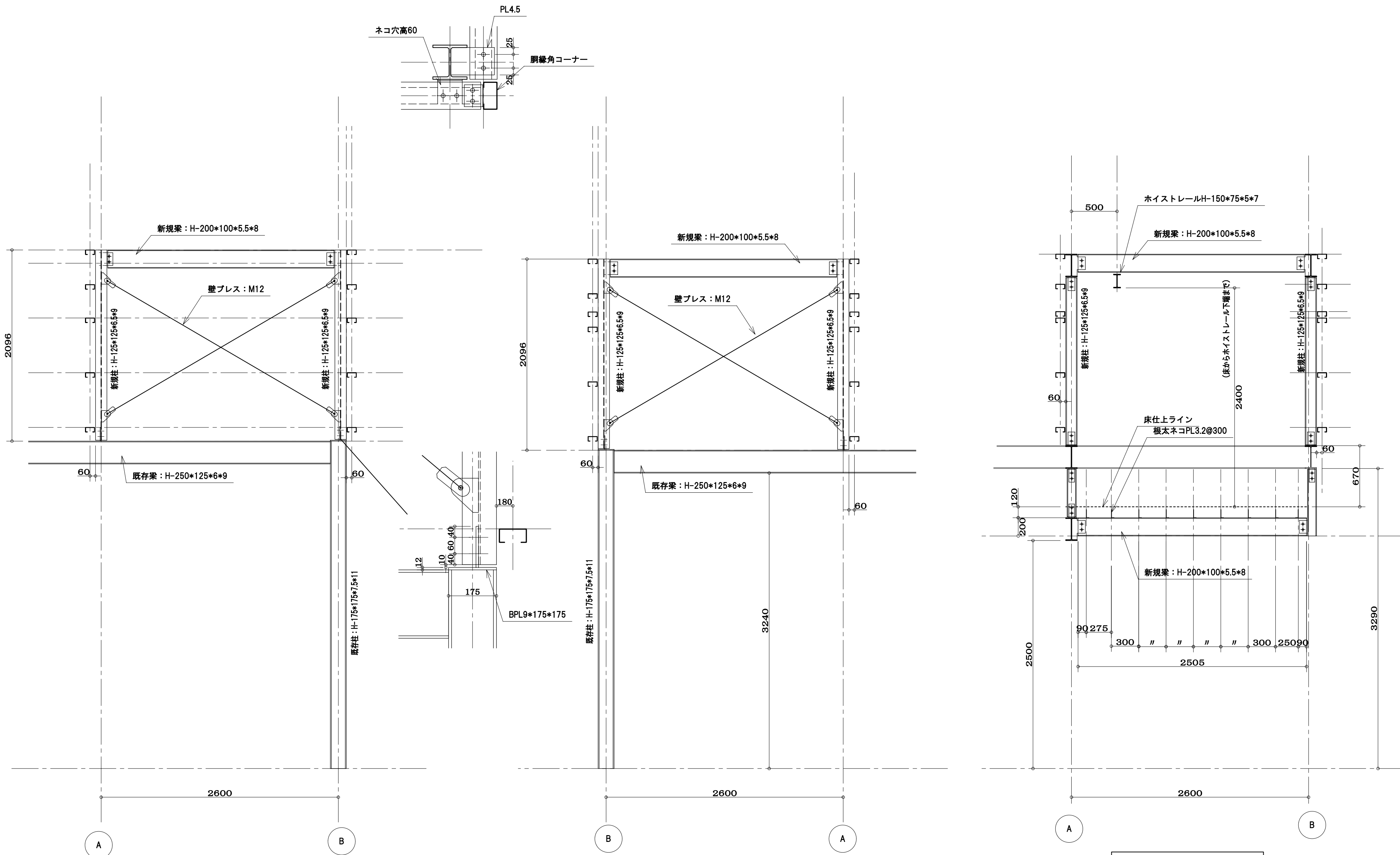
1 通鉄骨軸組図 S=1:30
